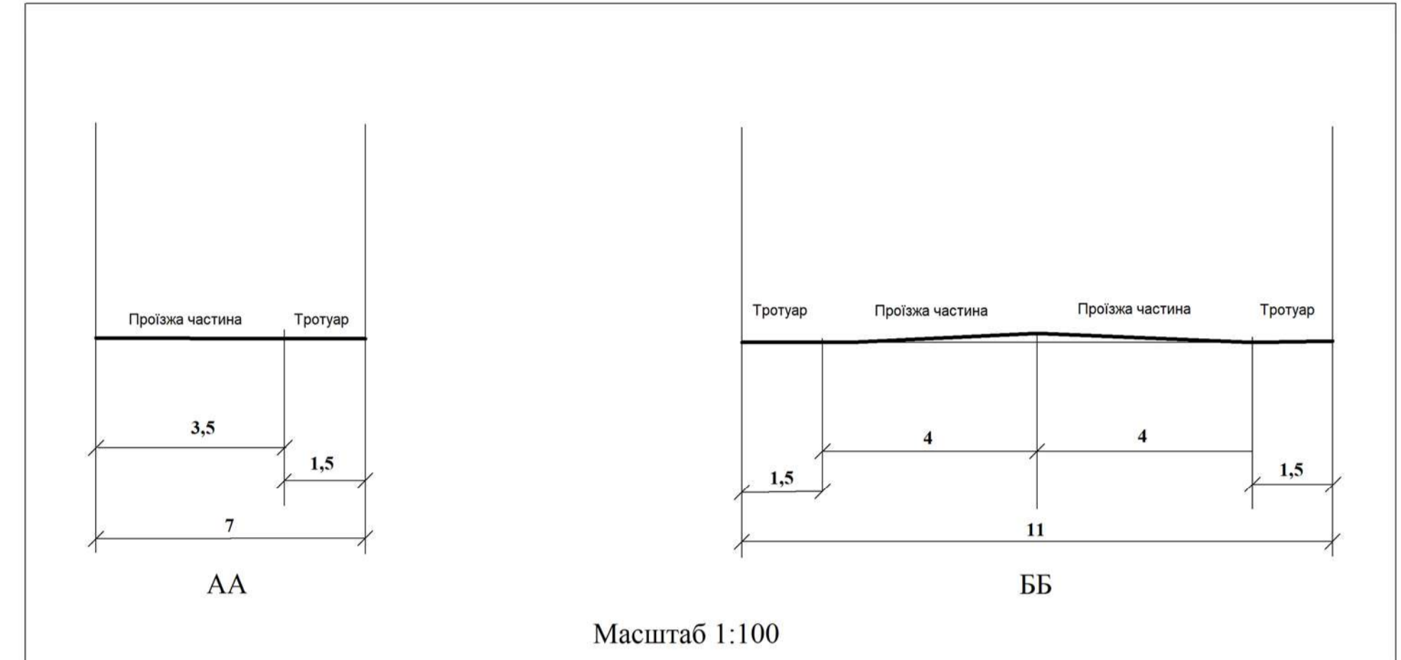
Поперечний профіль заїздів до ділянки (проектний)
